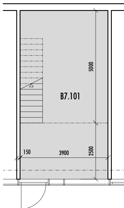
PÔDORYS 1.NP M 1:100
