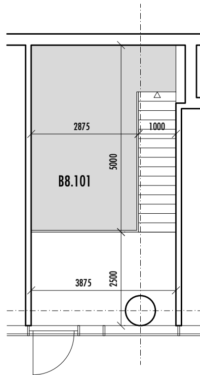
PÔDORYS HORNEJ ÚROVNE M 1:100
