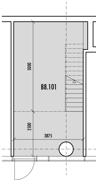
PÔDORYS 1.NP M 1:100
